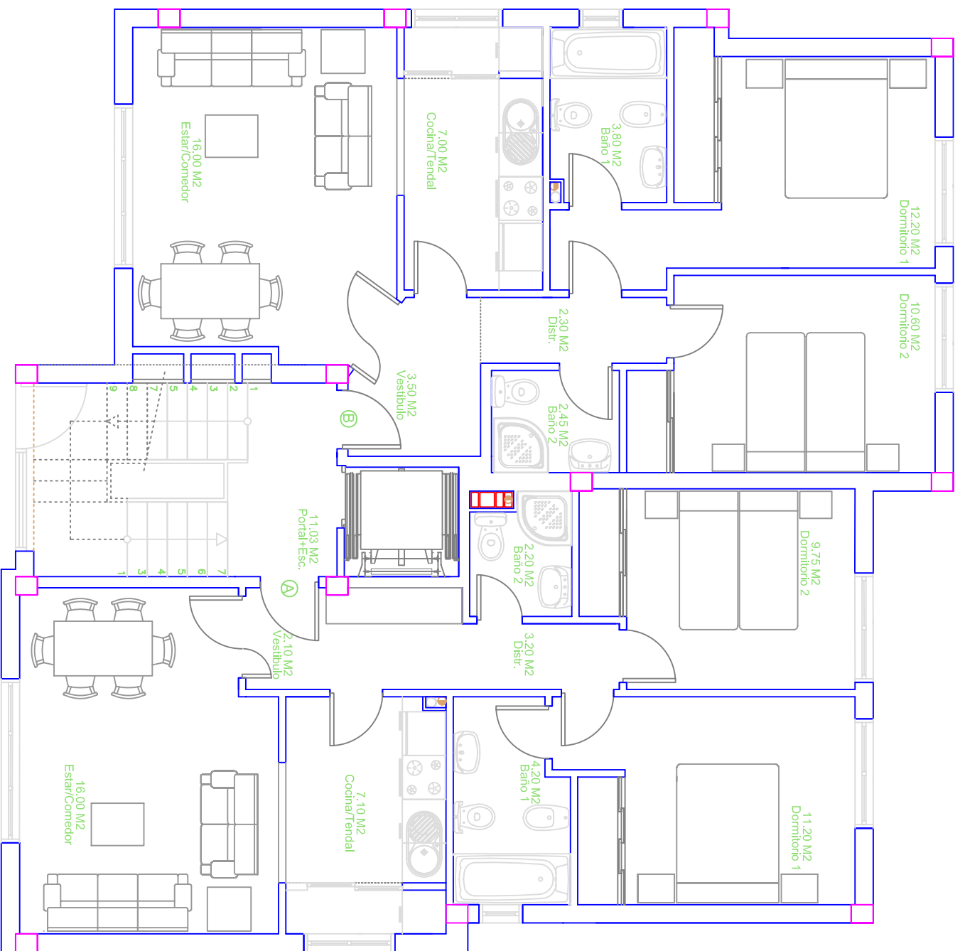
PLANTA BAJA BLOQUE TIPO
