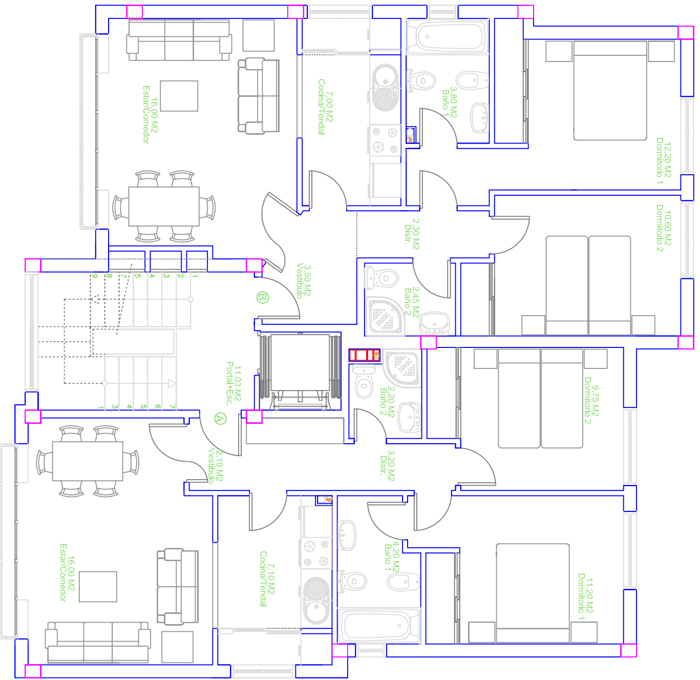
PLANTA PRIMERA BLOQUE TIPO
